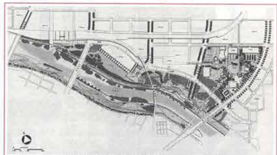
図-4 忠別川河川空間整備イメージ図
