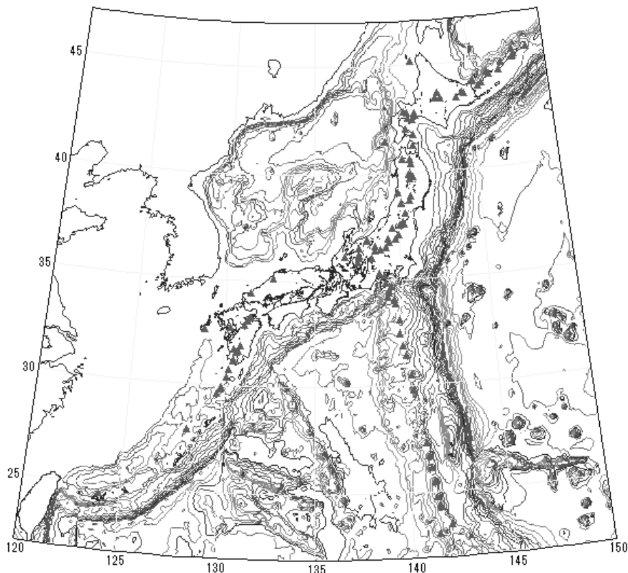
図1 日本列島周辺の海底地形、活火山、活断層の分布
